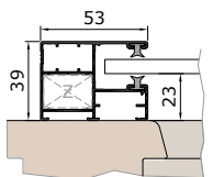
KF53V vezetősín
