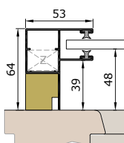
Termikusan leválasztott KD53VT vezetősín
