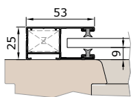
K53V vezetősín
