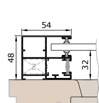
KR54V vezetősín
