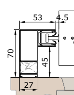
ED53V vezetősín
