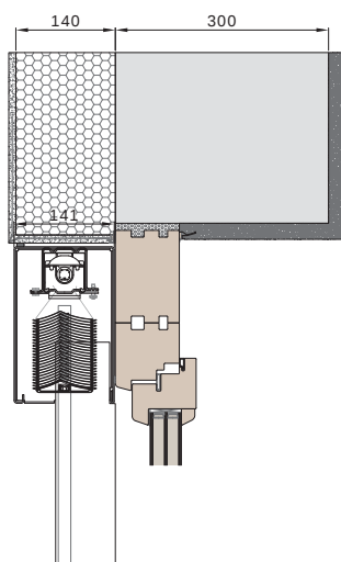
Hőszigetelő rendszerrel és tokmagasítással. RAFF S Blende.
