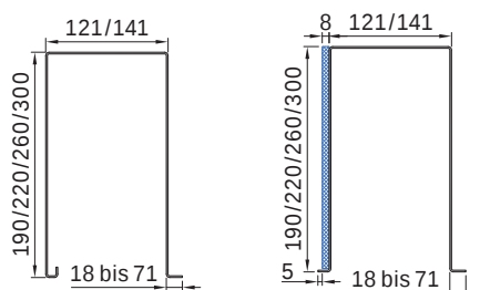
Nyílásnagyságok RAFF F
