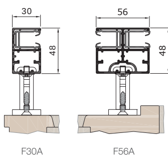
Vezetősínek RAFF A
